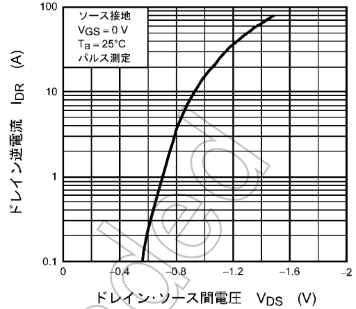
図 8.8 I_{DR} - V_{DS}
