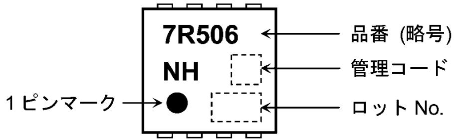
図 7.1 現品表示
