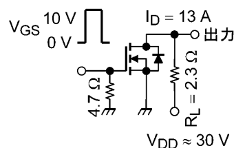
図 6.2.1 スwitchング時間の測定回路
