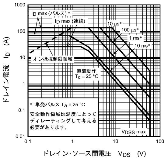
図 8.14 安全動作領域 (最大値 (保証値))
