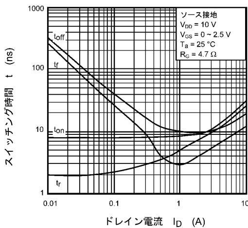
図 7.11 t - I_D
