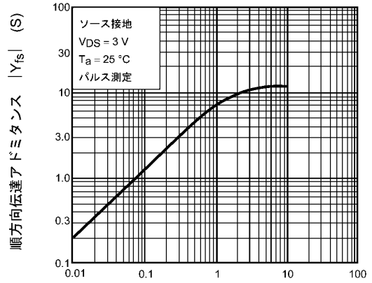
図 7.8 |Y_{fs}| - I_D
