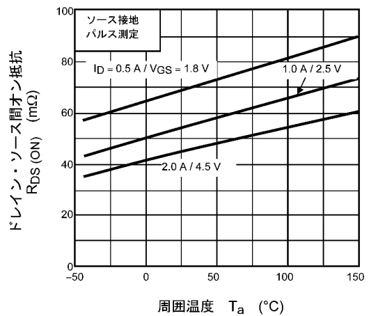
図 7.6 R_{DS(ON)} - T_a
