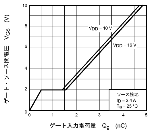
図 7.12 ダイナミック入力特性
