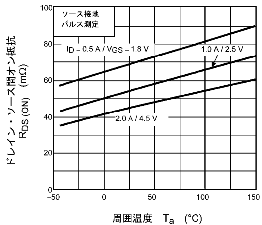
図 7.6 R_{DS(ON)} - T_a
