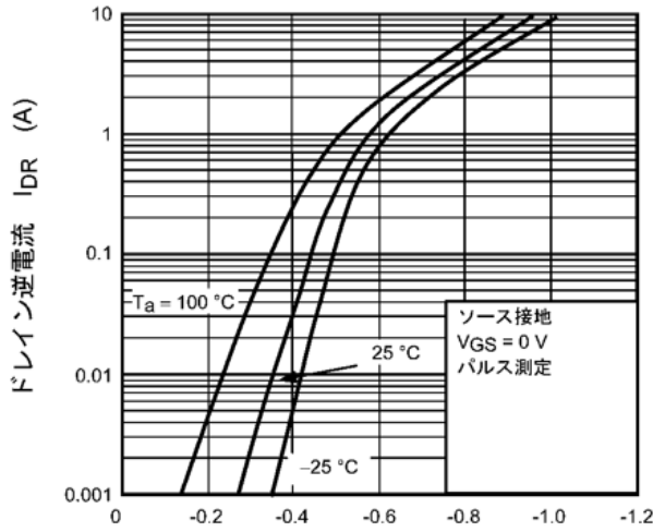
図 7.9 I_{DR} - V_{DS}
