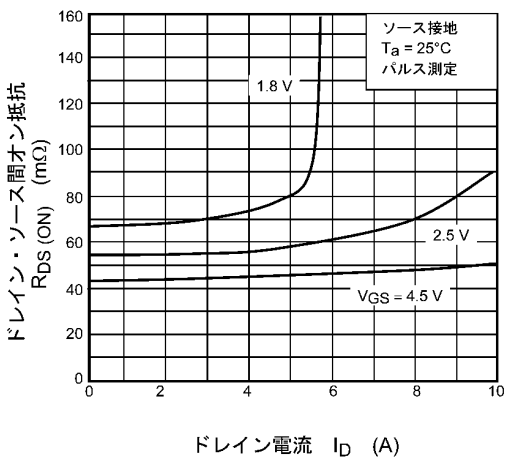
図 7.5 R_{DS(ON)} - I_D
