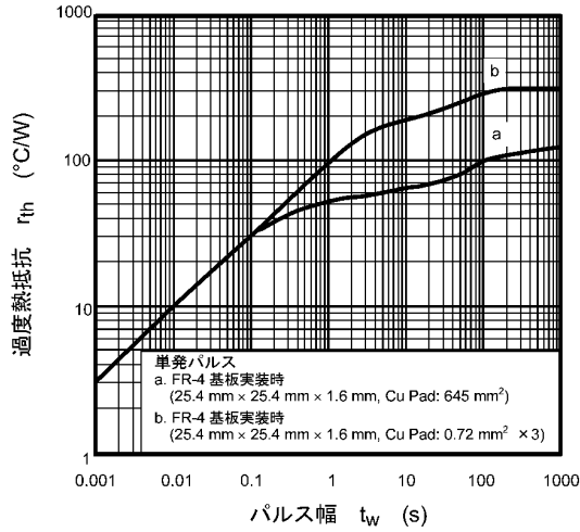
図 7.13 r_{th} - t_w
