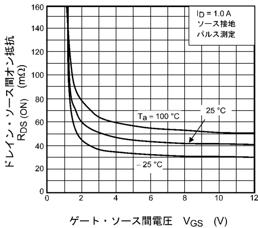
図 7.3 R_{DS(ON)} - V_{GS}
