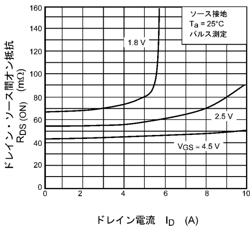
図 7.5 R_{DS(ON)} - I_D
