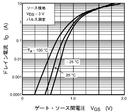
図 7.2 I_D - V_{GS}
