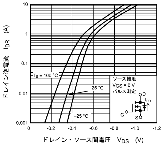
図 7.9 I_{DR} - V_{DS}
