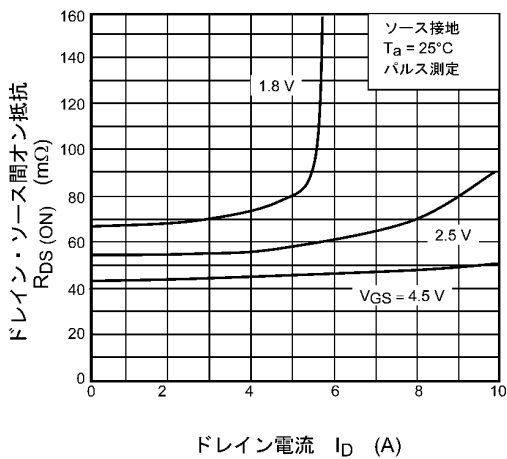
図 7.5 R_{DS(ON)} - I_D
