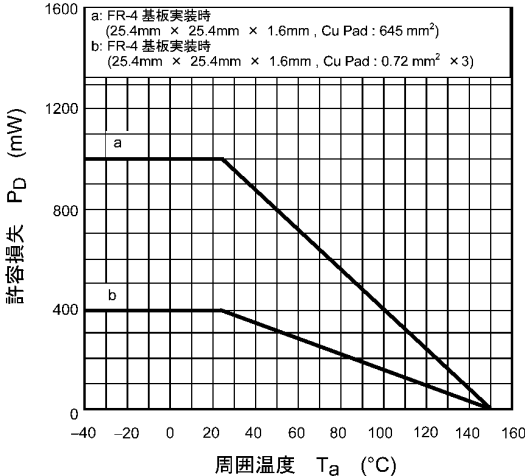
図 7.13 P_D - T_a
