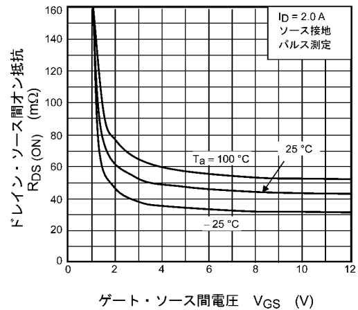
図 7.4 R_{DS(ON)} - V_{GS}
