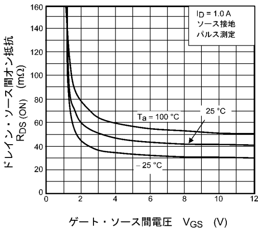
図 7.3 R_{DS(ON)} - V_{GS}
