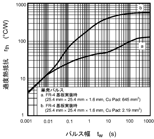
図 7.13 r_{th} - t_w
