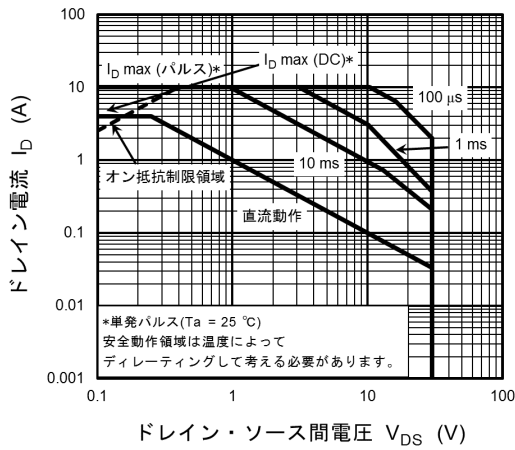
図 7.15 安全動作領域
