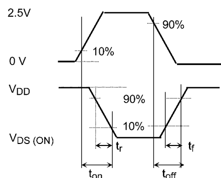
図 5.3.2 入力波形/出力波形
