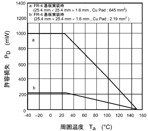
図 7.14 P_D - T_a
