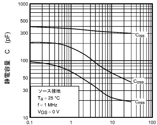
図 7.10 C - V_{DS}
