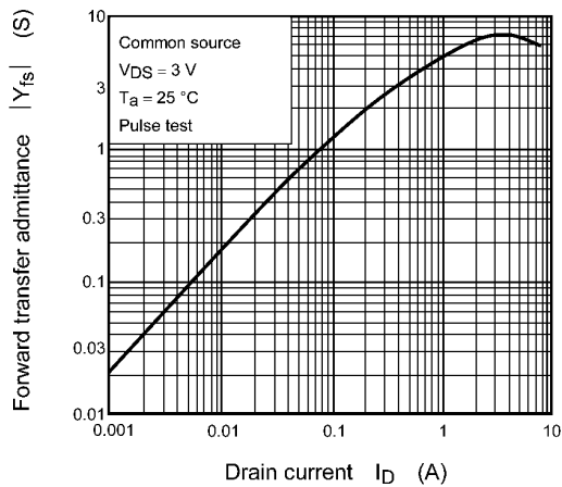
Fig. 9.8 |Y_{fs}| - I_D
