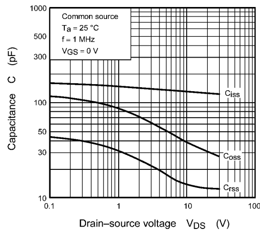
Fig. 9.10 C - V_{DS}
