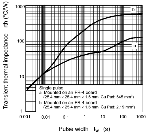
Fig. 9.13 r_{th} - t_w
