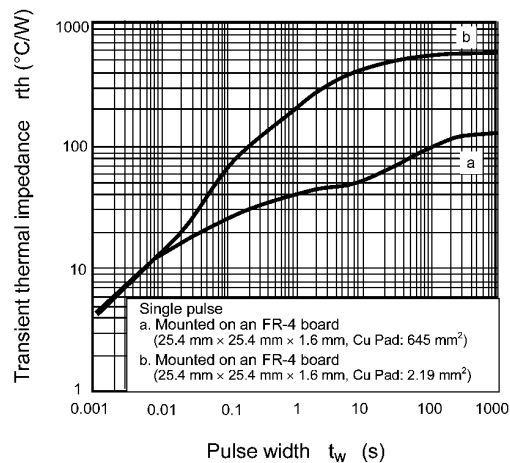
Fig. 9.13 r_{th} - t_w
