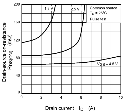
Fig. 9.5 R_{DS(ON)} - I_D
