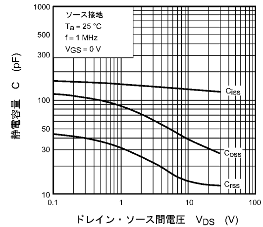
図 9.10 C - V_{DS}
