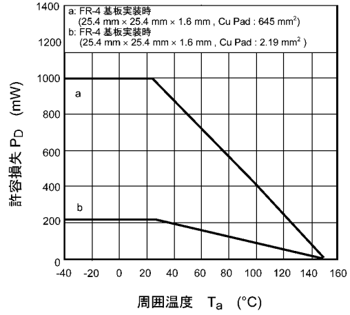
図 7.14 P_D - T_a
