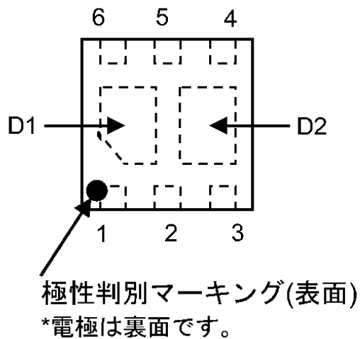
図 6.2 ピン配置(Top View)
