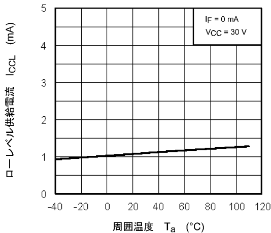
図 12.2.6 I_{CCL} - T_a
