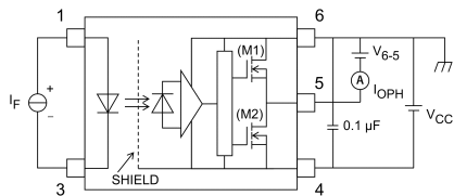
図 12.1.1 I OPH 測定回路
