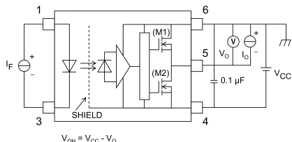
図 12.1.3 V OH 測定回路
