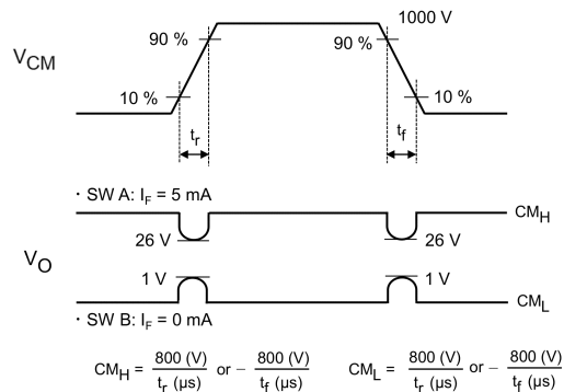
図 12.1.8 コモンモードノイズ除去電圧測定回路, 波形
