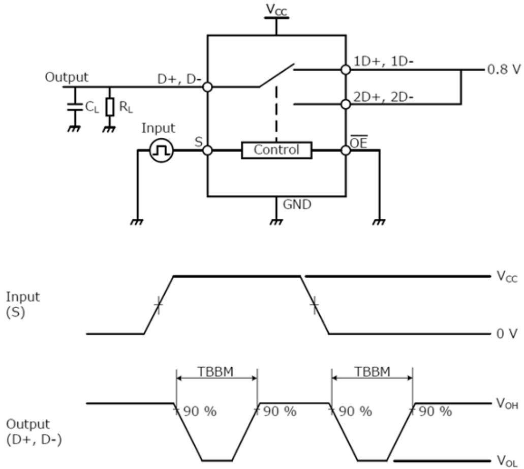
図 11.3 ブレーク・ビフォー・メイク (TBBM)
