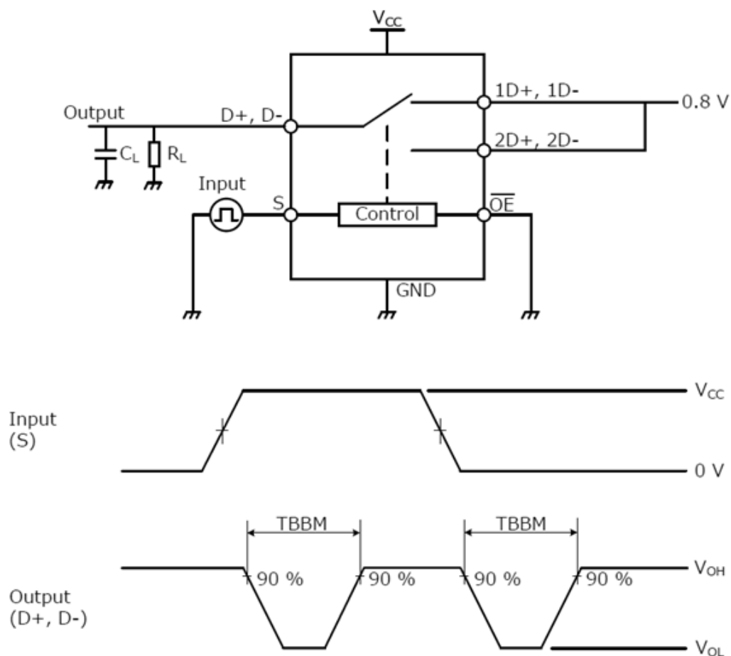
図 11.3 ブレーク・ビフォー・メーカー (TBBM)
