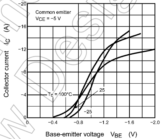
Fig. 8.4 I_c - V_{be}
