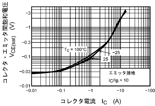
図 8.1 I_C - V_{CE}
