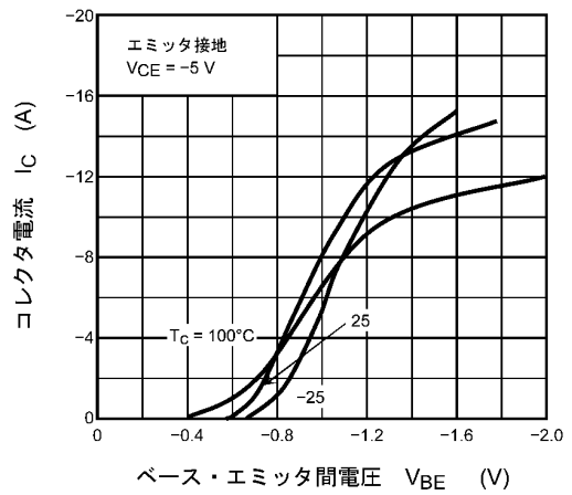
図 8.4 I_C - V_{BE}
