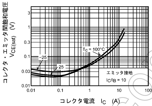
図 8.1 I_C - V_{CE}
