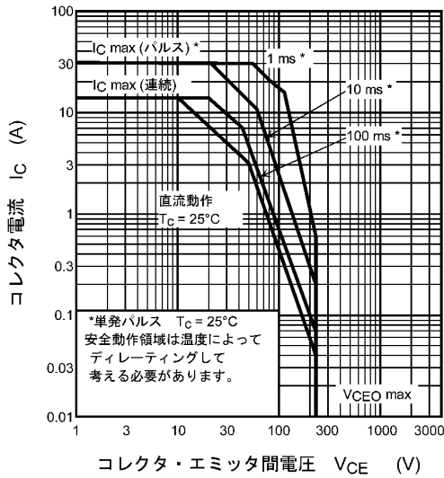
図 8.6 安全動作領域 (最大値 (保証値))
