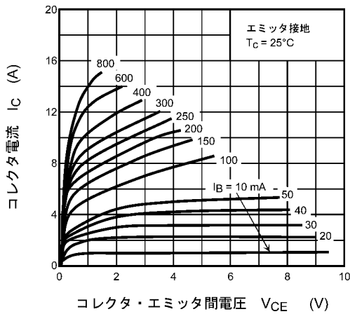
図 8.1 I_C - V_{CE}
