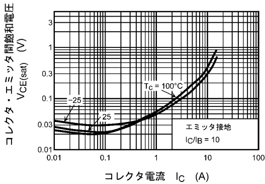
図 8.1 I_C - V_{CE}
