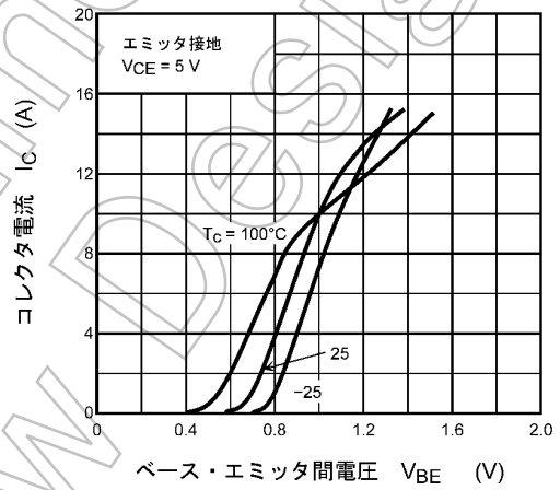
図 8.4 I_C - V_{BE}
