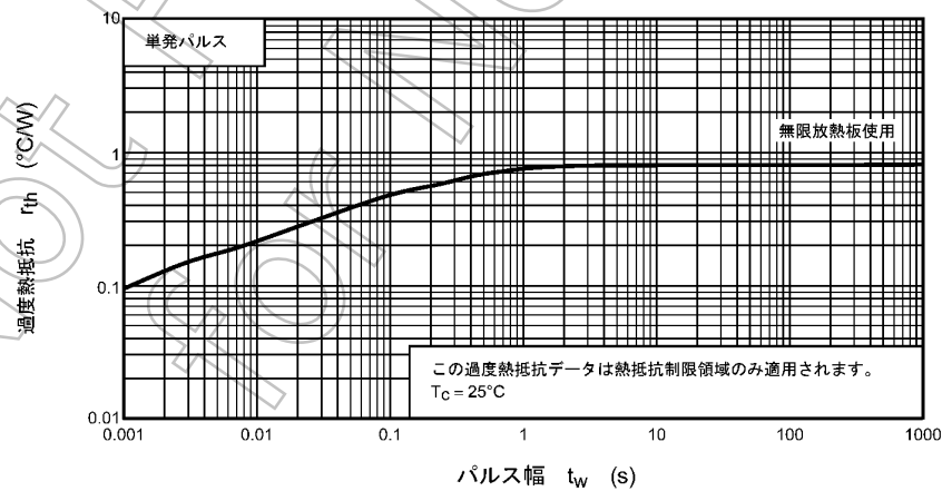
図 8.5 r_{th(j-c)} - t_w (最大値 (保証値))
