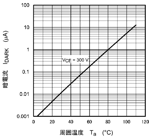
図 11.11 I_{DARK} - T_a
