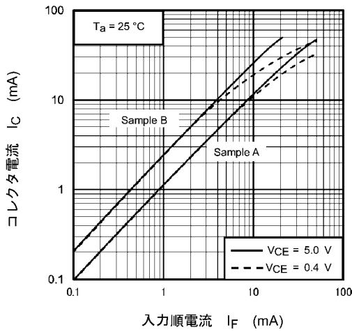
図 11.9 I_C - I_F
