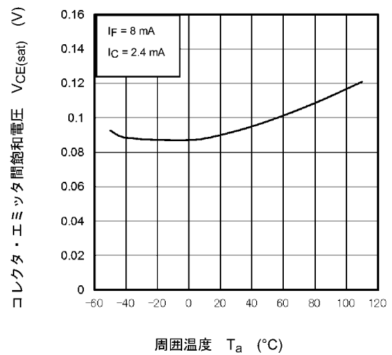
図 11.12 V_{CE(sat)} - T_a
