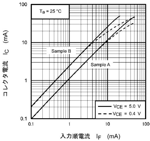
図 11.9 I_C - I_F
