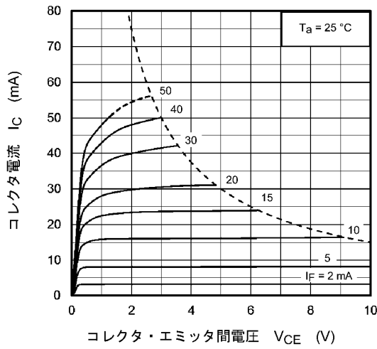
図 11.7 I_C - V_{CE}
