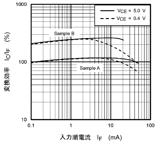
図 11.10 I_C/I_F - I_F
