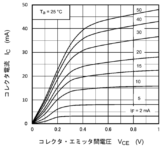
図 11.8 I_C - V_{CE}
