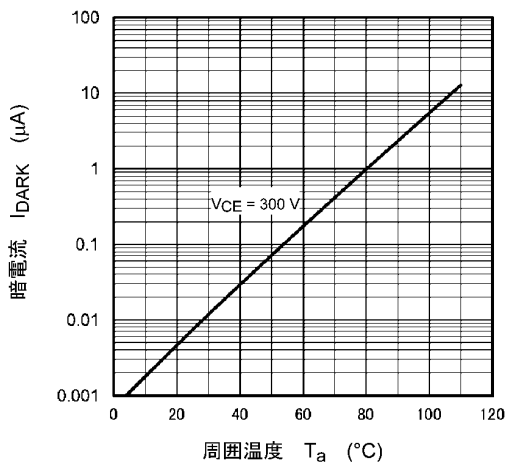
図 11.11 I_{DARK} - T_a
