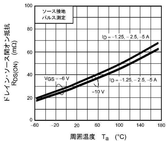
図 8.6 R_{DS(ON)} - T_a (注8)
