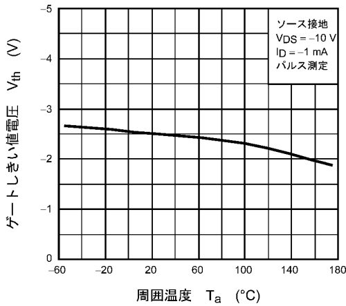
図 8.9 V_{th} - T_a (注8)
