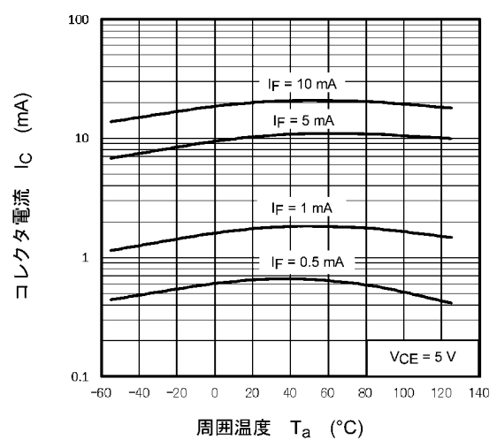
図 11.12 I_C - T_a
