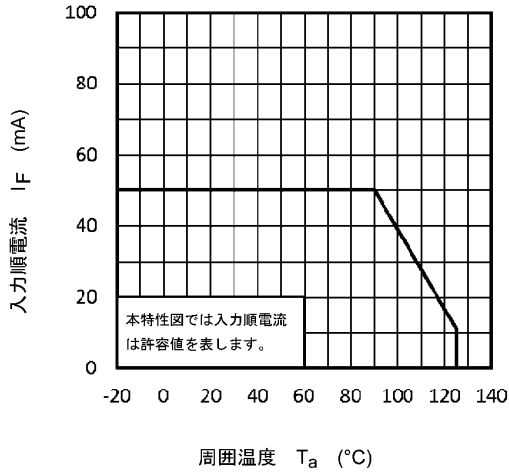
図 11.1 I_F - T_a
