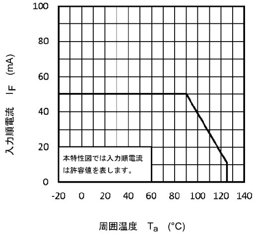
図 11.1 I_F - T_a
