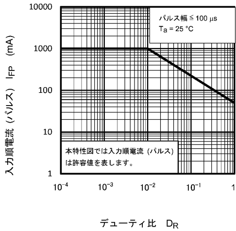
図 11.3 I_{FP} - D_R
