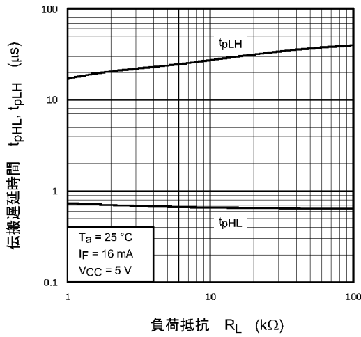
図 11.15 t_{pHL}, t_{pLH} - R_L
