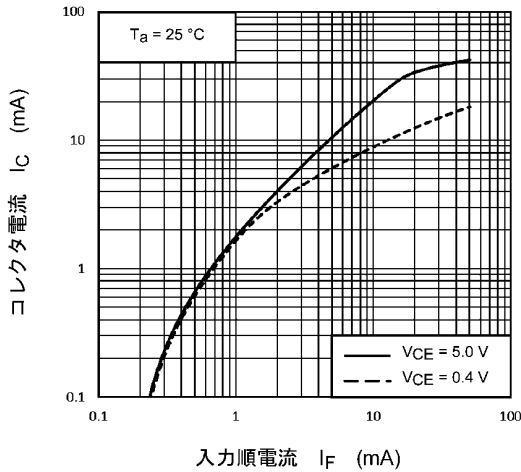
図 11.9 I_C - I_F
