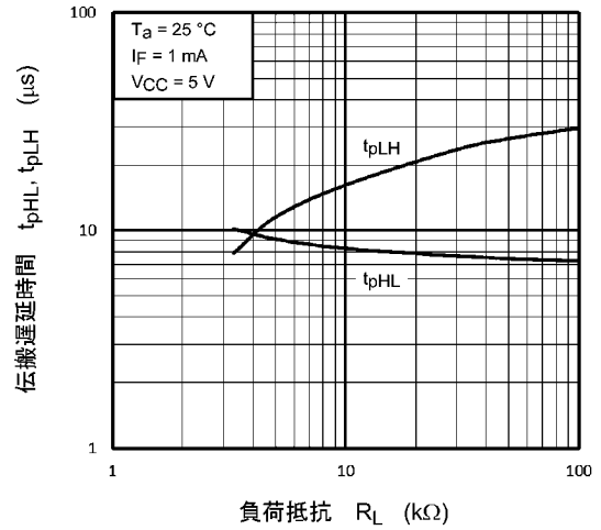
図 11.14 t_{pHL}, t_{pLH} - R_L
