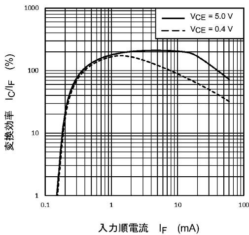
図 11.11 I_C/I_F - I_F
