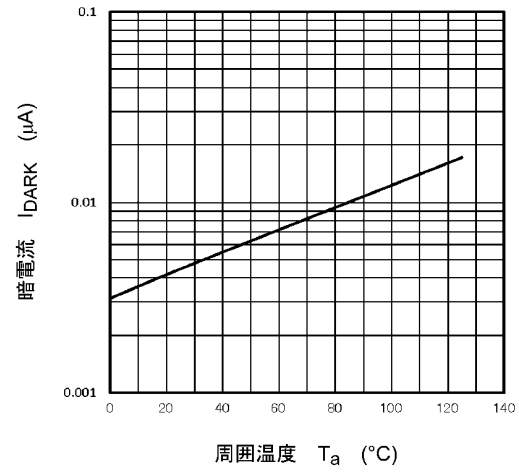
図 11.10 I_{\text{DARK}} - T_a
