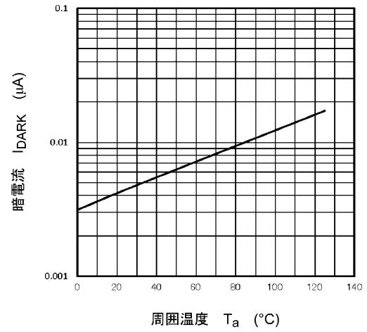
図 11.10 I_{DARK} - T_a
