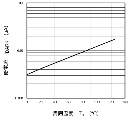
図 11.10 I_{DARK} - T_a
