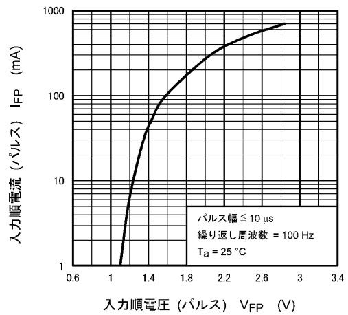
図 11.6 I_{FP} - V_{FP}
