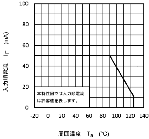
図 11.1 I_F - T_a
