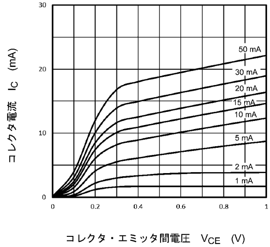
図 11.8 I_C - V_{CE}
