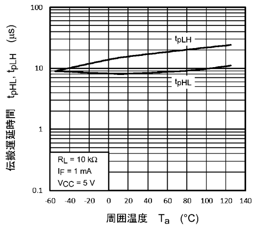
図 11.16 t_{pHL}, t_{pLH} - T_a
