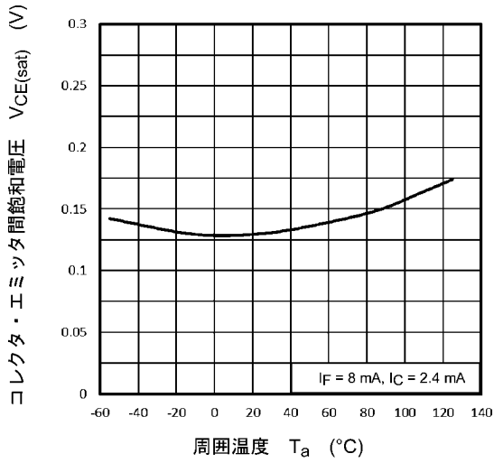
図 11.13 V_{CE(sat)} - T_a
