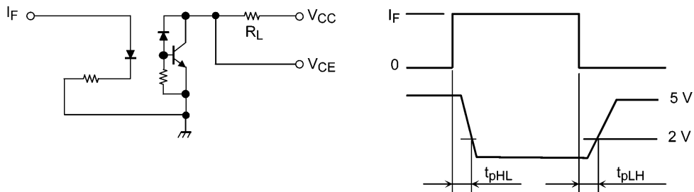
図 10.1 伝搬遅延時間測定回路, 波形
