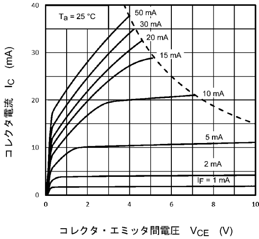
図 11.7 I_C - V_{CE}
