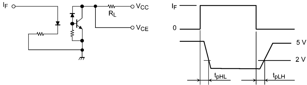
図 10.1 伝搬遅延時間測定回路
