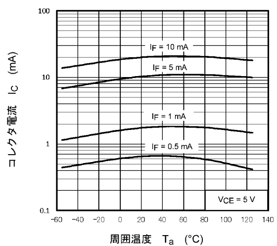
図 11.12 I_C - T_a
