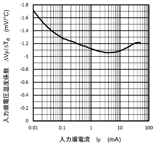
図 11.5 \Delta V_F / \Delta T_a - I_F
