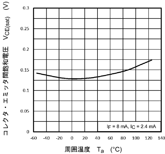
図 11.13 V_{CE(sat)} - T_a
