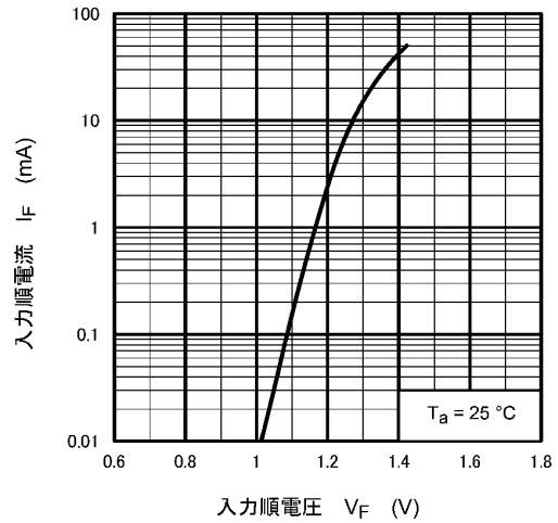
図 11.4 I_F - V_F
