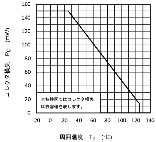
図 11.2 P_C - T_a
