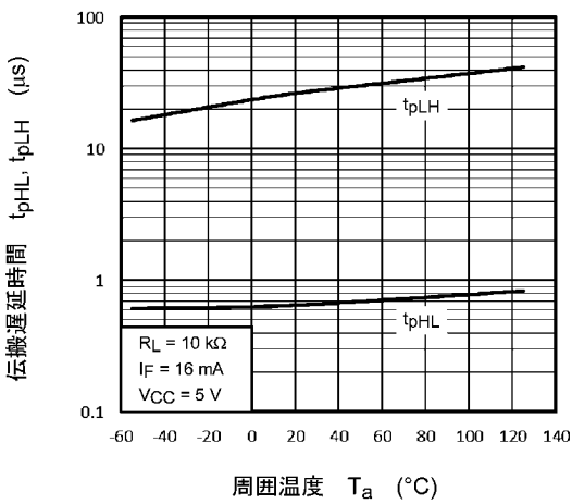
図 11.17 t_{pHL}, t_{pLH} - T_a
