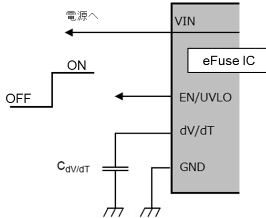
UVLO 端子の接続例 (外部制御)
