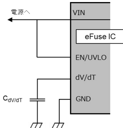
EN/UVLO 端子の接続例 (VIN 直結)
