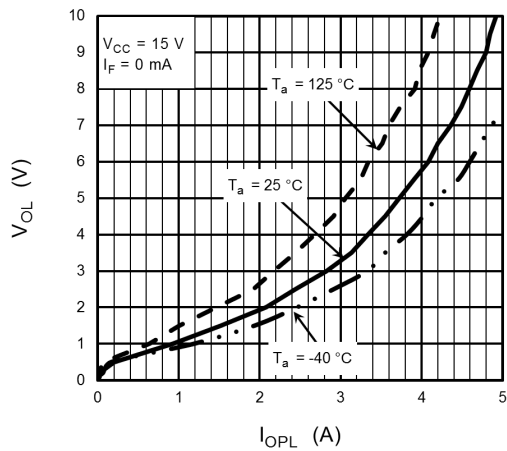
图 13.2.9 V_{OL} - I_{OPL}
