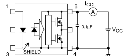
図 13.1.6 ICCL測定回路
