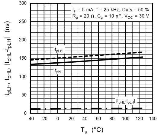
図 13.2.14 t_{pLH}, t_{pHL}, |t_{pHL} - t_{pLH}| - T_a
