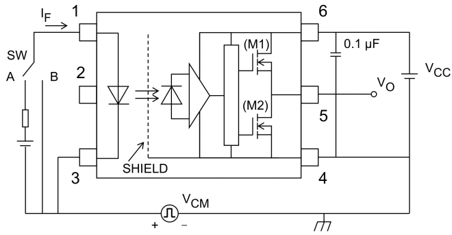
図 13.1.9 コモンモード過渡耐性測定回路, 波形
