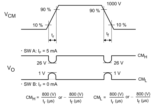
図 13.1.9 コモンモード過渡耐性測定回路, 波形
