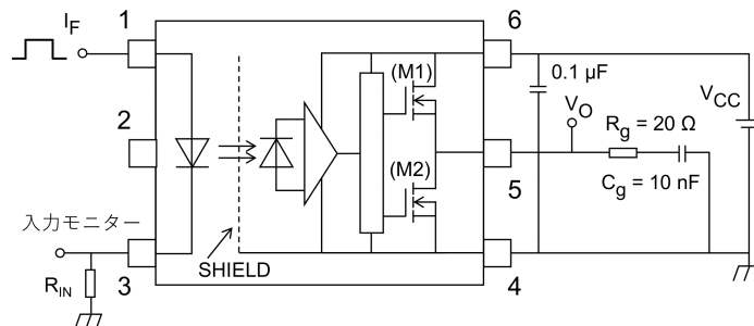
図 13.1.8 伝搬遅延時間測定回路, 波形
