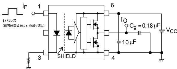
図 13.1.7 IOLH / IOHL測定回路
