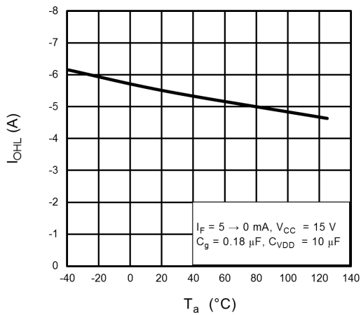
图 13.2.11 I_{OHL} - T_a
