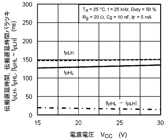
図 13.2.16 t_{pLH}, t_{pHL}, |t_{pHL} - t_{pLH}| - V_{CC}
