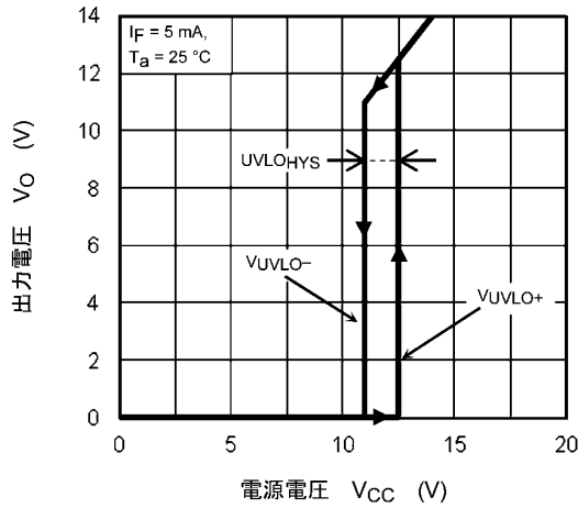
図 13.2.13 V_O(V_{UVLO}) - V_{CC}
