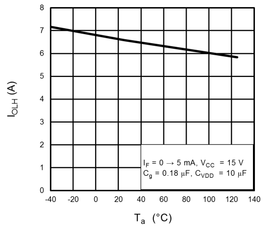
图 13.2.12 I_{OLH} - T_a
