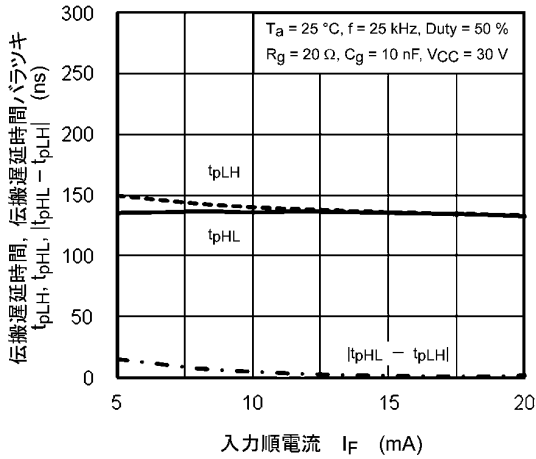
図 13.2.15 t_{pLH}, t_{pHL}, |t_{pHL} - t_{pLH}| - I_F
