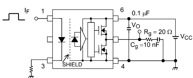
図 13.1.8 伝搬遅延時間測定回路, 波形
