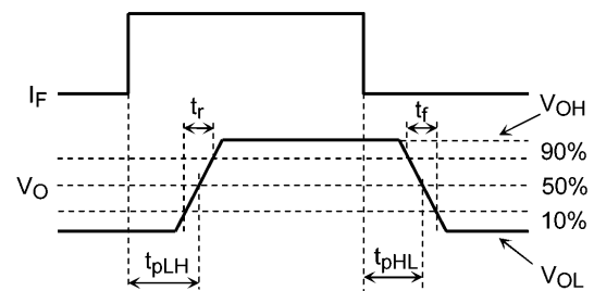
図 13.1.8 伝搬遅延時間測定回路, 波形
