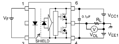
図 13.1.4 VOL測定回路
