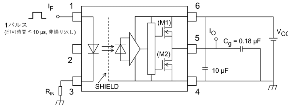
図 13.1.7 I OLH / I OHL 測定回路
