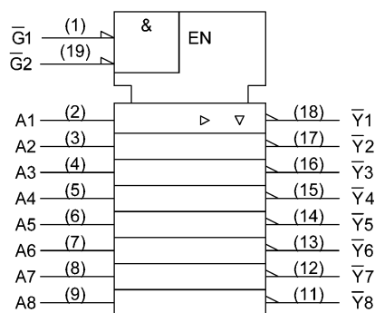
TC74ACT540FT
