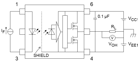
Fig. 13.1.3 V_{OH} Test Circuit
