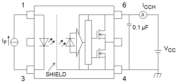
Fig. 13.1.5 I_{CCH} Test Circuit
