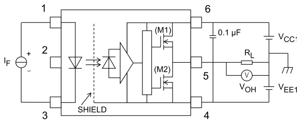
Fig. 13.1.3 V_{OH} Test Circuit
