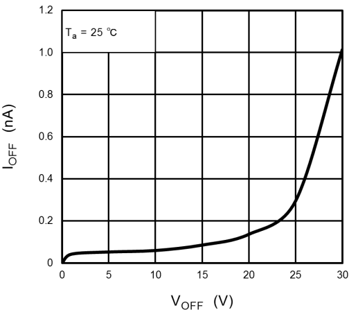
Fig. 12.8 I_{OFF} - V_{OFF}
