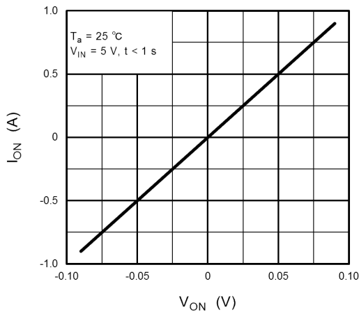
Fig. 12.3 I_{ON} - V_{ON}
