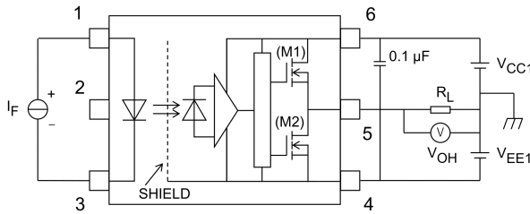
図 13.1.3 V OH 測定回路
