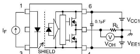
图 13.1.3 V OH 测定回路
