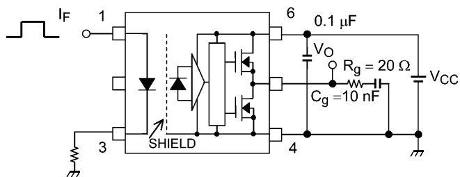
图 13.1.7 伝搬遅延時間測定回路, 波形
