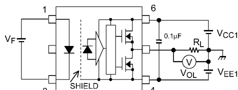
图 13.1.4 V OL 测定回路
