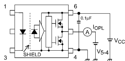
图 13.1.2 I OPL 测定回路
