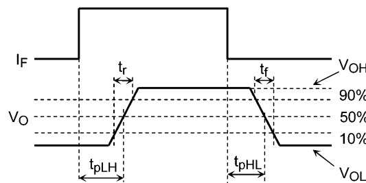
图 13.1.7 伝搬遅延時間測定回路, 波形
