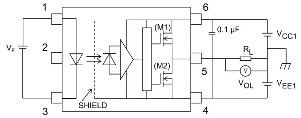
図 13.1.4 V OL 測定回路
