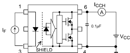
图 13.1.5 I CCH 测定回路
