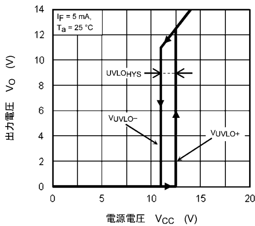
図 13.2.11 V_o(V_{UVLO}) - V_{CC}
