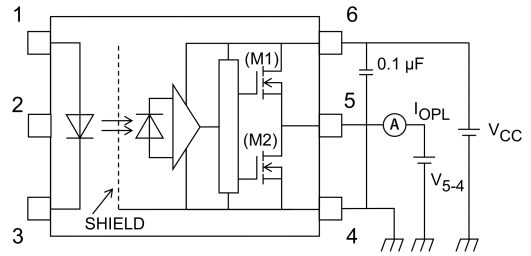
図 13.1.2 I OPL 測定回路
