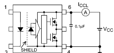
图 13.1.6 I CCL 测定回路
