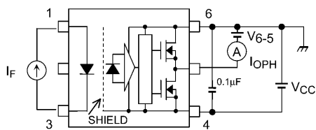
图 13.1.1 I OPH 测定回路
