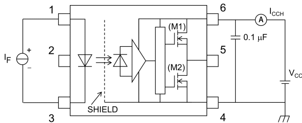
図 13.1.5 I CCH 測定回路
