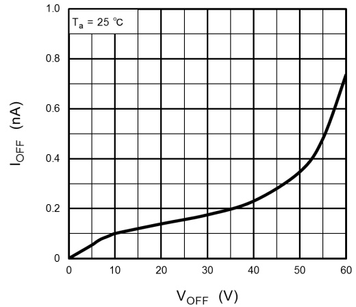
Fig. 12.8 I_{OFF} - V_{OFF}
