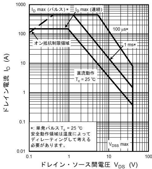
図 8.20 安全動作領域 (最大値 (保証値))
