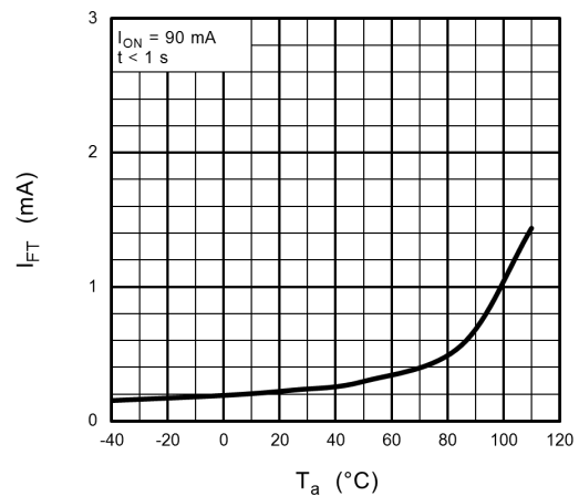
図 14.6 I_{FT} - T_a
