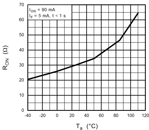
図 14.5 R_{ON} - T_a
