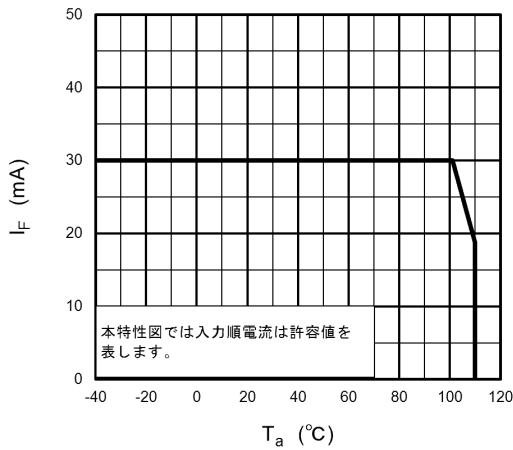
図 14.1 I_F - T_a
