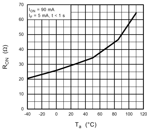
図 14.5 R_{ON} - T_a
