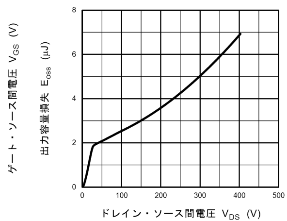
図 8.12 E_{oss} - V_{DS}
