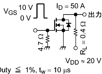
図 6.2.1 スwitching時間の測定回路
