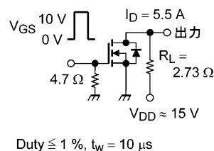
図 6.2.1 スwitching時間の測定回路例
