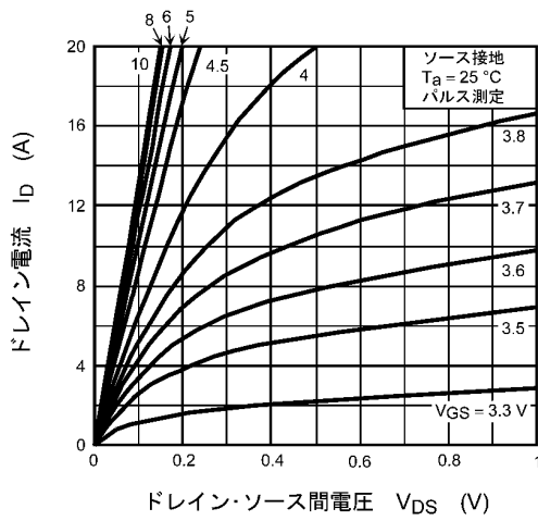
図 8.1 I_D - V_{DS}
