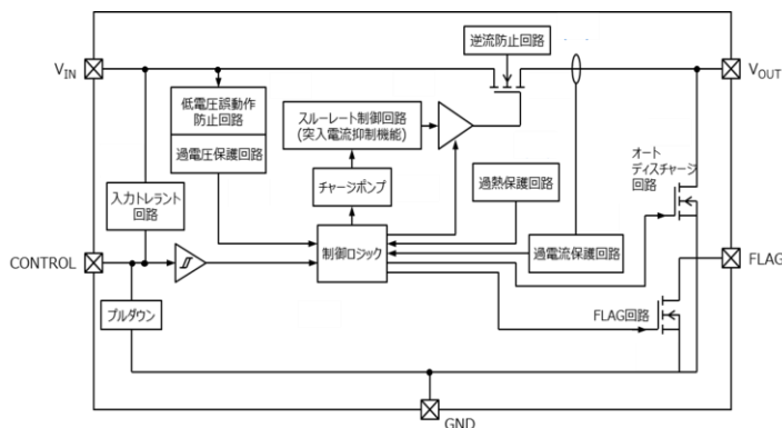
ロードスイッチIC ブロック図例
