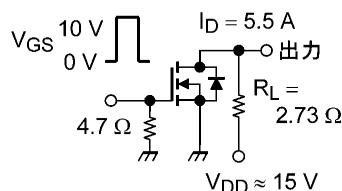
図 6.2.1 スwitching時間の測定回路例
