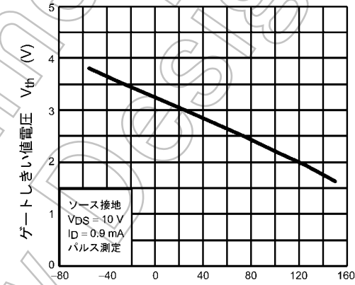
図 8.10 V_{th} - T_a
