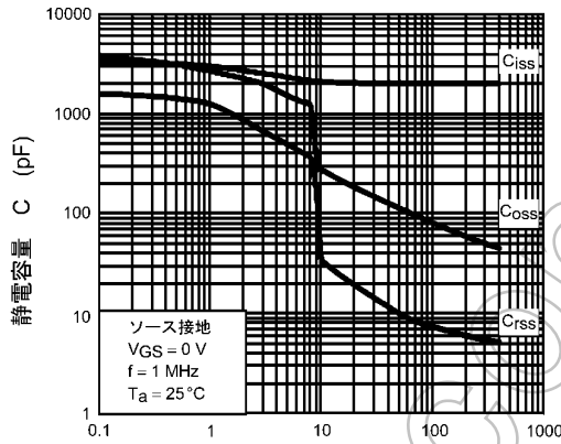
図 8.9 C - V_{DS}
