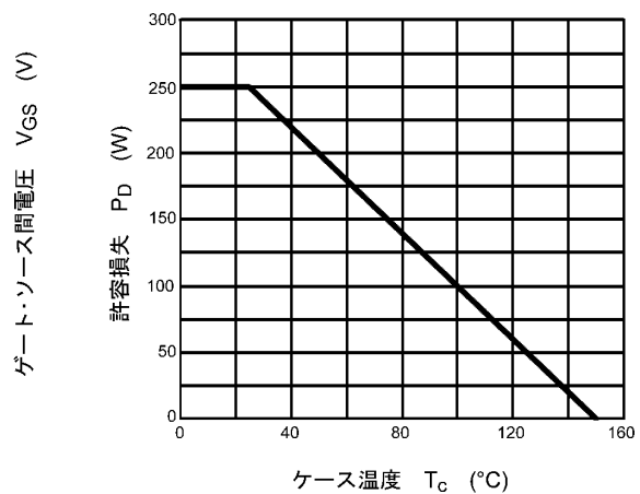
図 8.12 P_D - T_c (最大値 (保証値))
