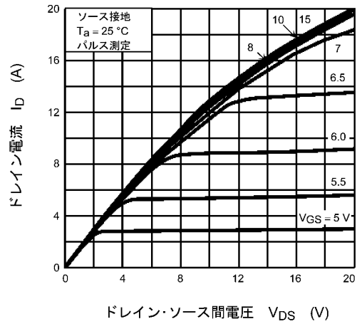
図 8.2 I_D - V_{DS}
