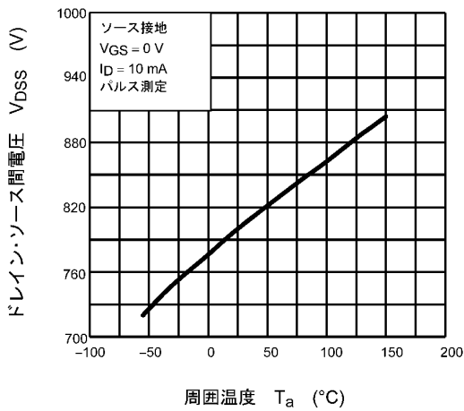
図 8.5 V_{DS} - T_a
