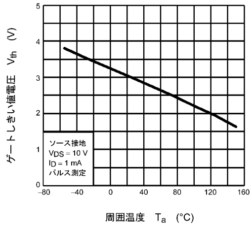
図 8.10 V_{th} - T_a
