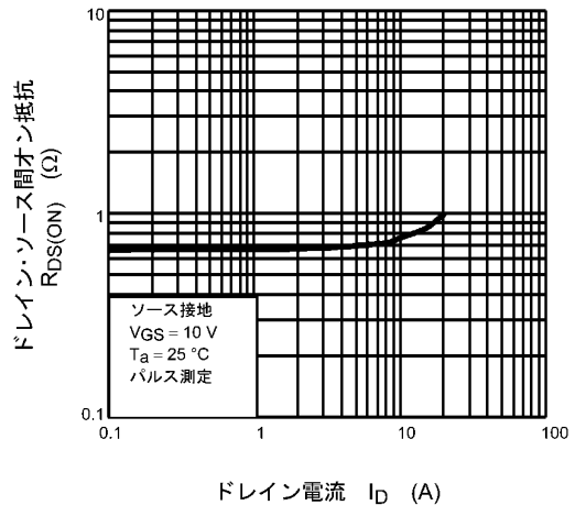
図 8.6 R_{DS(ON)} - I_D
