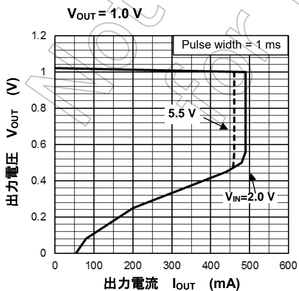
出力電圧—出力電流例
