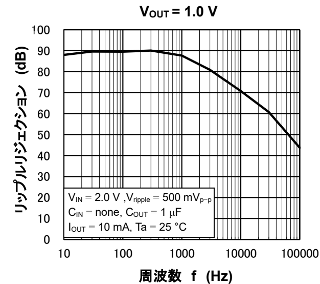
リップル除去率—周波数特性代表例
