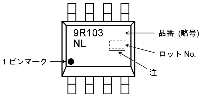
図 7.1 現品表示
