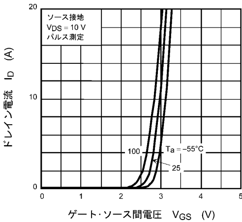
図 8.3 I_D - V_{GS}
