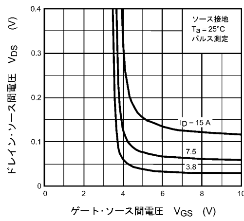
図 8.4 V_{DS} - V_{GS}
