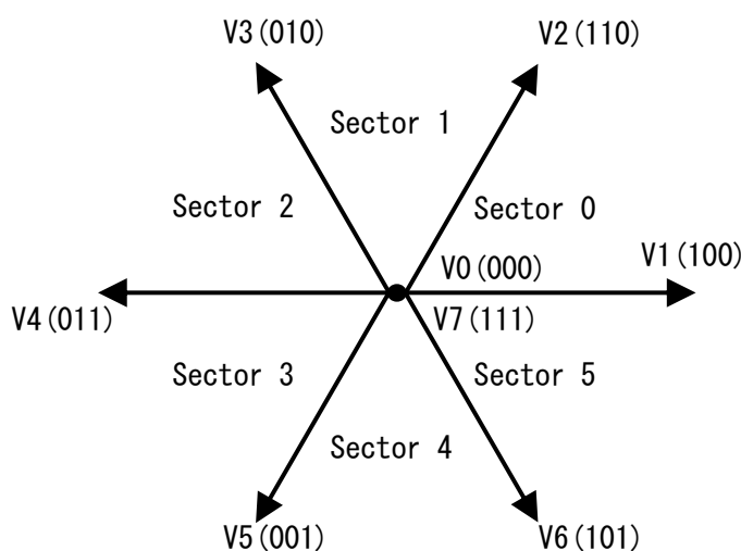
図 9.11 空間ベクトル
