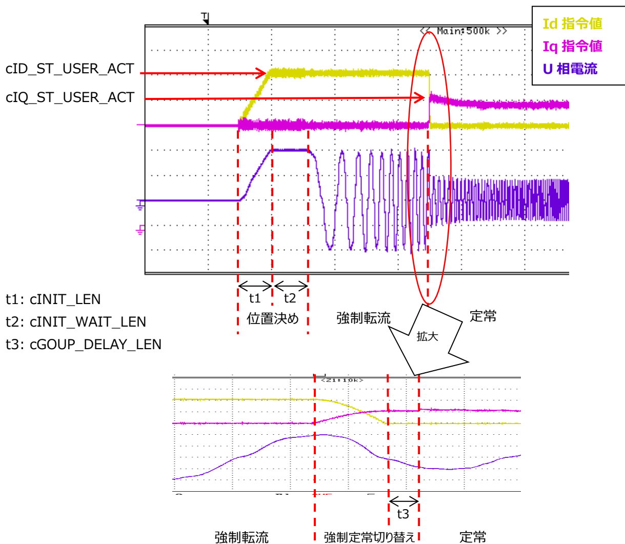
図 10.1 始動電流波形(電気角 0°に位置決め)
