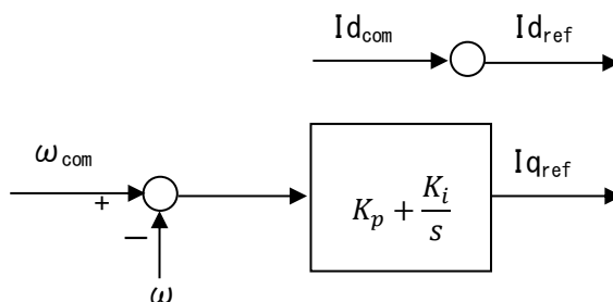
図 9.9 速度制御ブロック図
