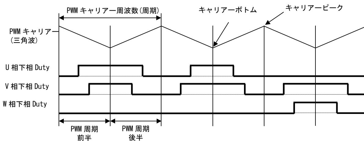
図 9.4 2相変調の場合
