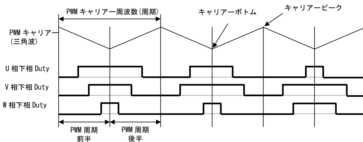
図 9.3 3相変調の場合
