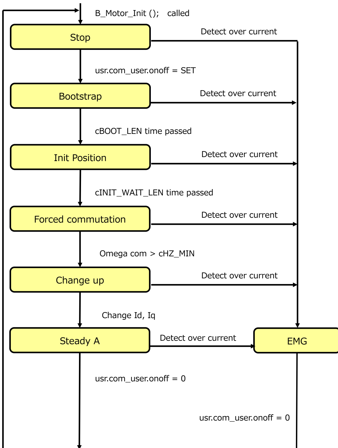
図 7.1 モーター動作の状態遷移
