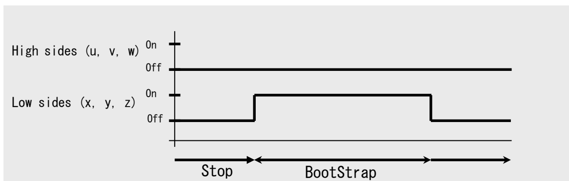
図 9.2 ブートストラップ時間
