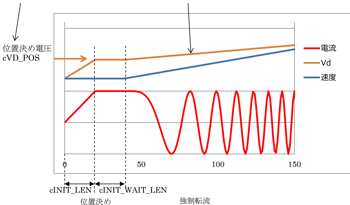
図 10.2 電圧駆動時のパラメータ調整方法
