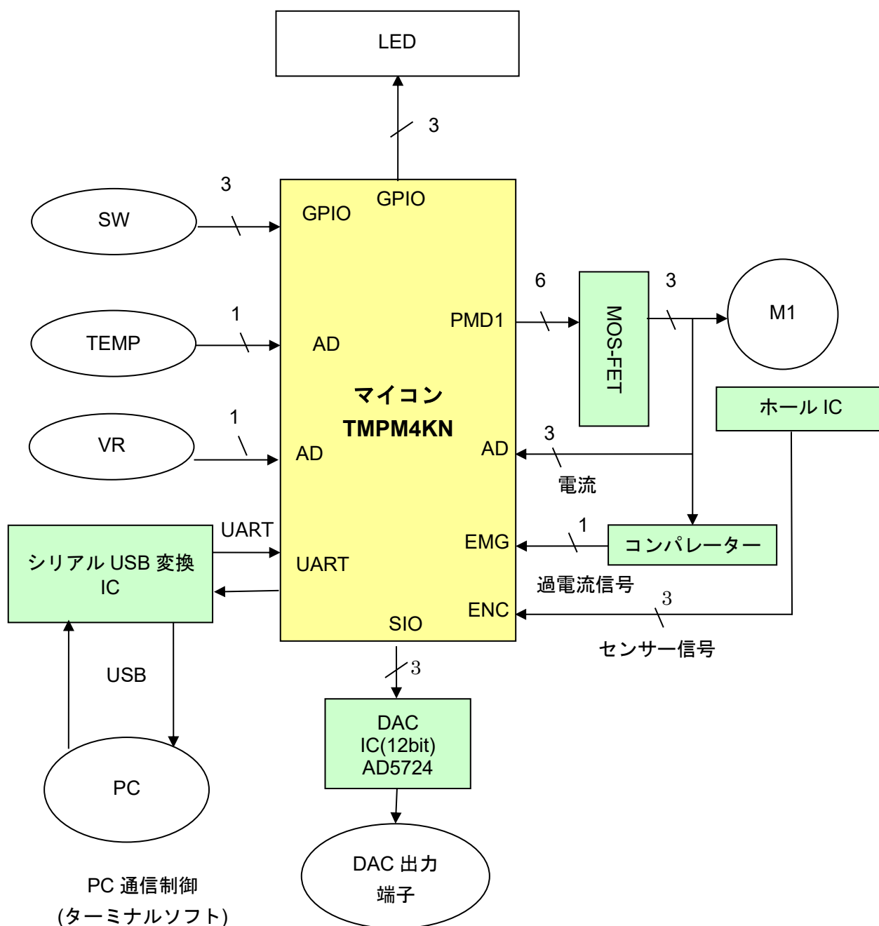
図 2.1 システムブロック図
