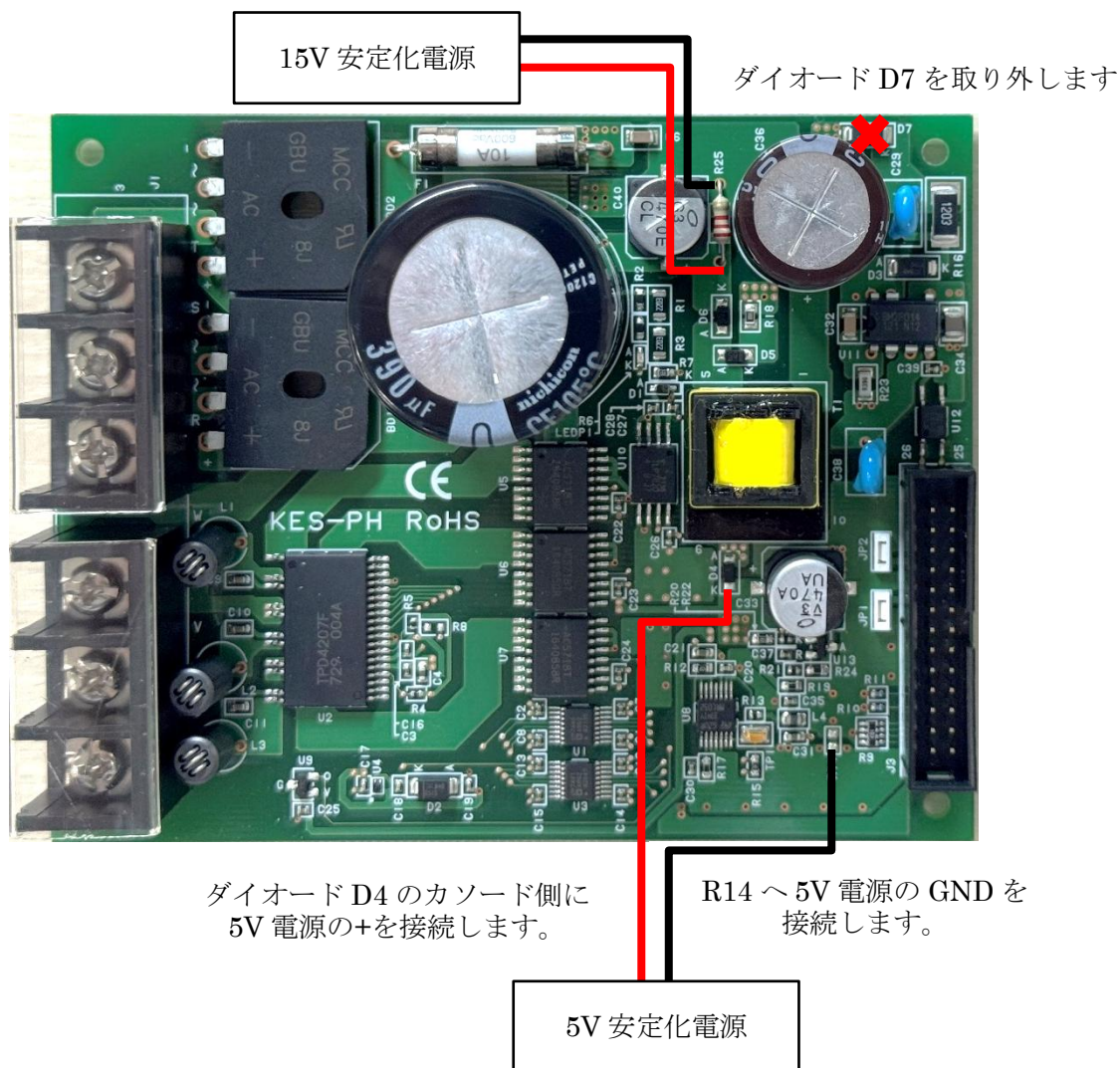
図 1.4 基板修正(KES-PH)
