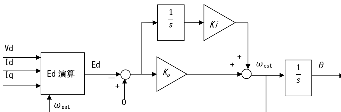
図 9.7 d 軸誘起電圧 E_d による位置推定ブロック図
