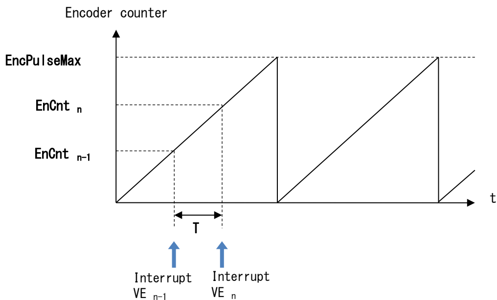
図 9.8 エンコーダーパルスからの位置および速度演算
