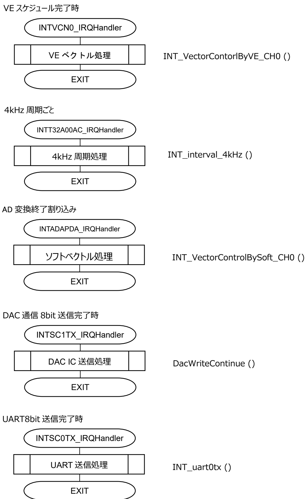
図 6.3 割り込み
