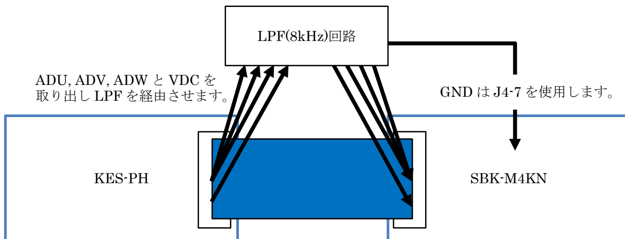
図 1.3 LPF の追加
