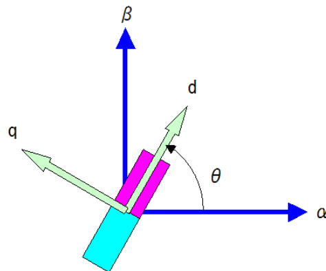
図 9.6 パーク変換
