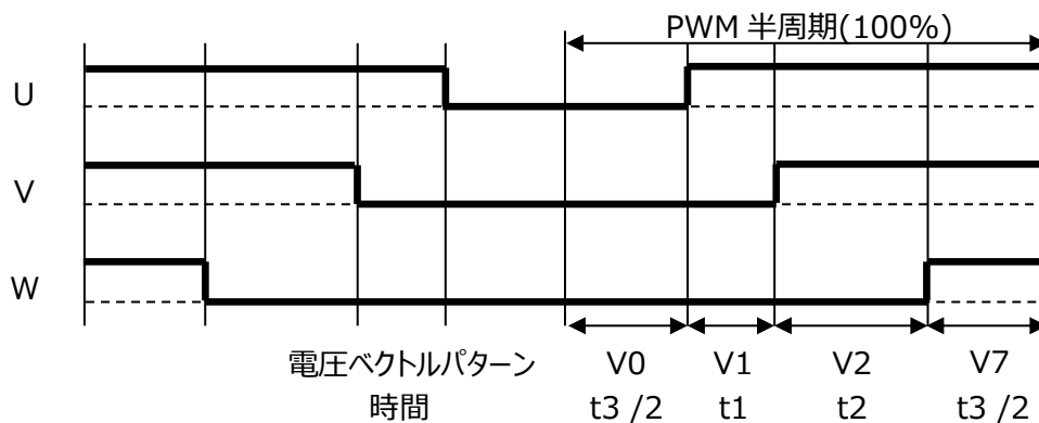
図 9.13 3 相変調時の PWM 波形
