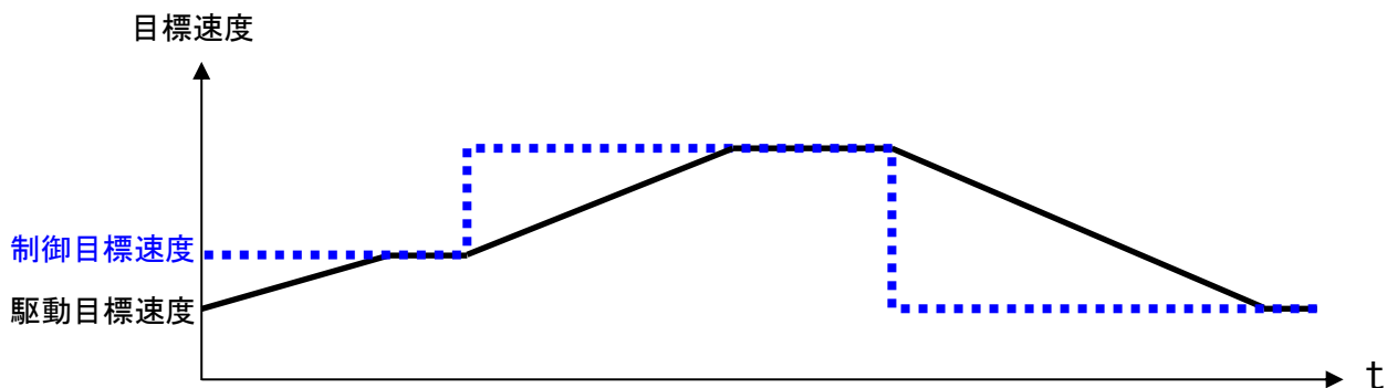
図 1.2 制御目標速度と駆動目標速度
