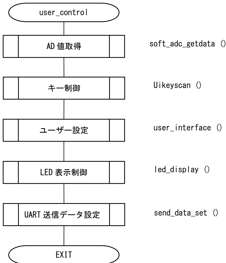
図 8.1 ユーザー制御
