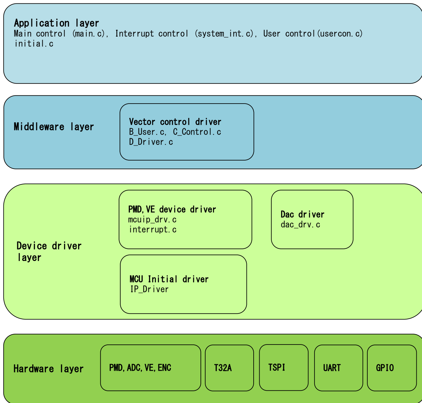
図 4.1 モジュール構成
