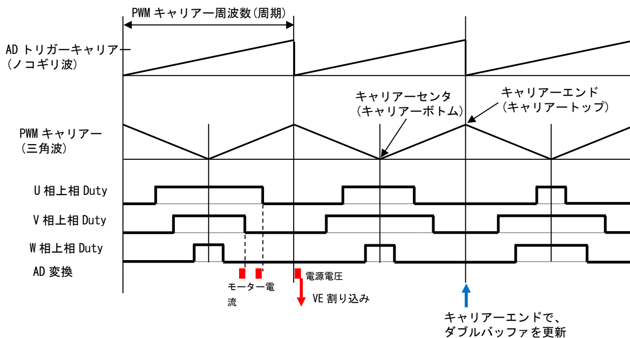
図 11.2 1 シャント制御
