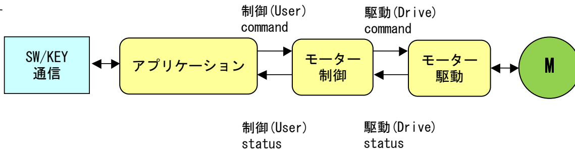
図 1.1 ベクトル制御ソフトウェアの構造
