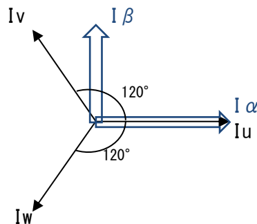
図 9.5 クラーク変換
