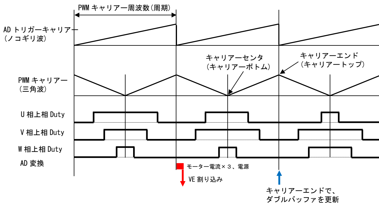
図 11.1 3 シャント制御
