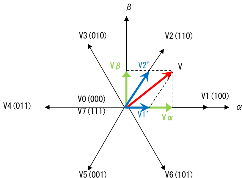
図 9.12 セクター0 時の電圧ベクトル
