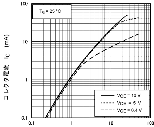
図 11.9 I_C - I_F
