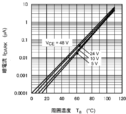
図 11.11 I_{\text{DARK}} - T_a
