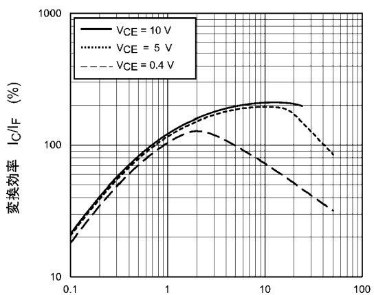
図 11.10 I_C/I_F - I_F
