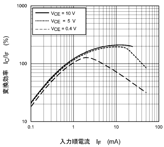
図 11.10 I_C/I_F - I_F
