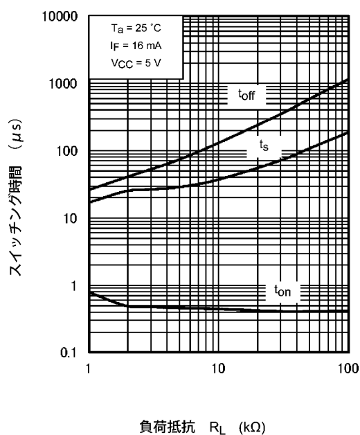
図 11.14 スイッチング時間 - R_L
