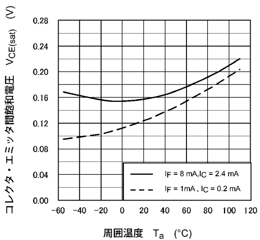
図 11.12 V_{CE(\text{sat})} - T_a
