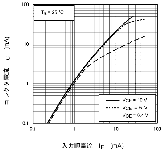
図 11.9 I_C - I_F
