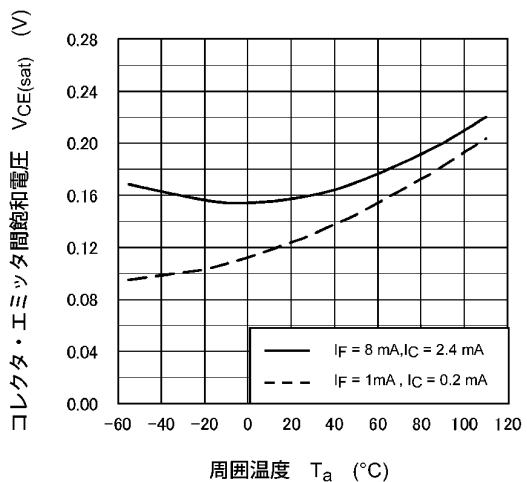
図 11.12 V_{CE(sat)} - T_a
