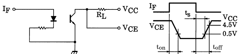
図 10.1 スイッチング測定回路, 波形
