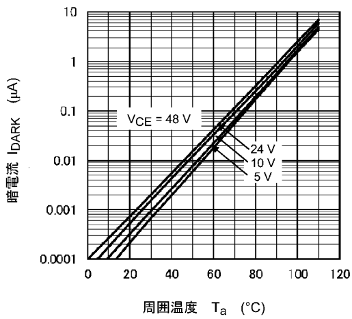
図 11.11 I_{DARK} - T_a
