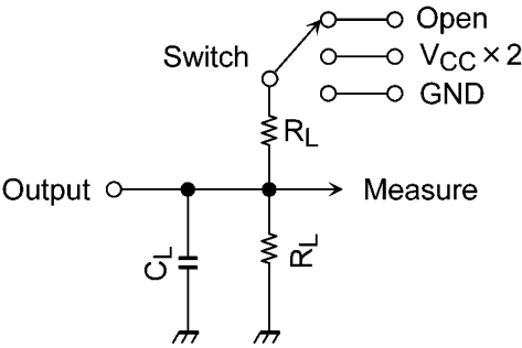
図 9.7.1 AC電気的特性測定回路
