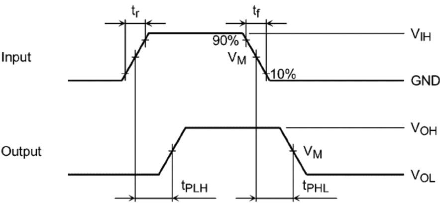
図 9.7.1 t_{PLH} , t_{PHL}
