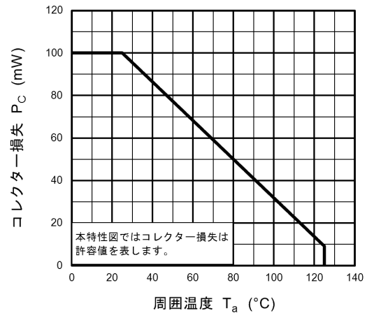
図 11.2 P_C - T_a
