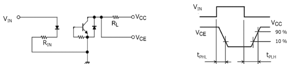
図 10.1 伝搬遅延時間測定回路, 波形
