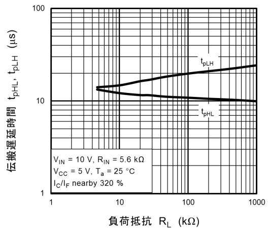
図 11.16 伝搬遅延時間 - R_L
