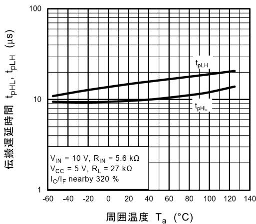
図 11.17 伝搬遅延時間 - T_a
