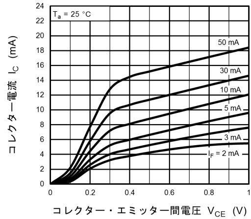
図 11.8 I_C - V_{CE}
