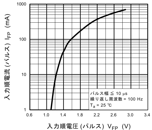
図 11.6 I_{FP} - V_{FP}
