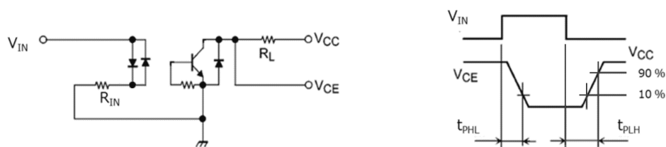
図 10.1 スイッチング時間測定回路, 波形
