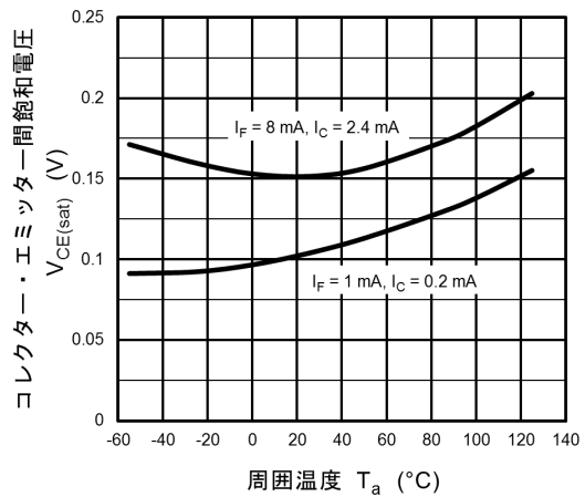
図 11.10 V_{CE(\text{sat})} - T_a
