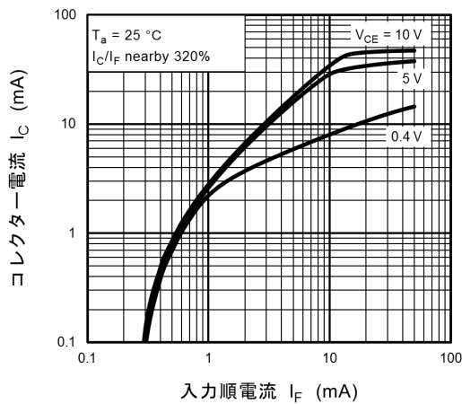
図 11.11 I_C - I_F
