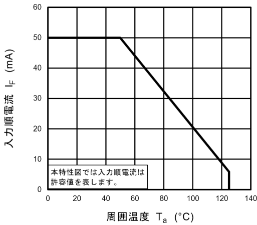
図 11.1 I_F - T_a
