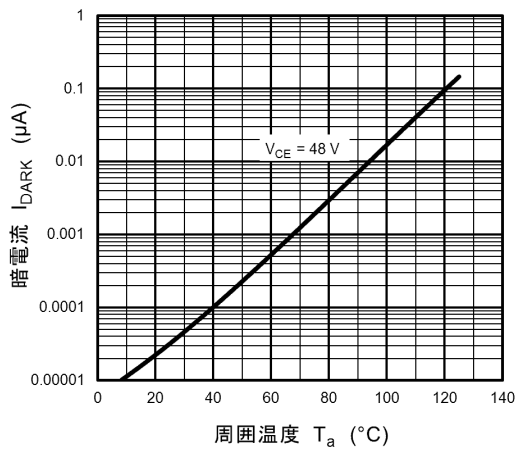
図 11.9 I_{\text{DARK}} - T_a
