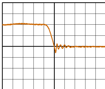
図 2.10 SBD リカバリー波形例
