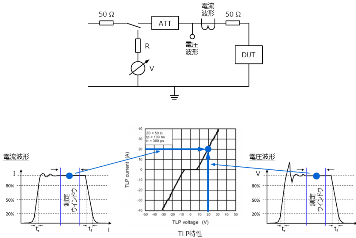
図 2.13 TLP 試験例
