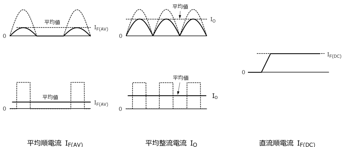
図 1.2 定常動作電流定格の定義
