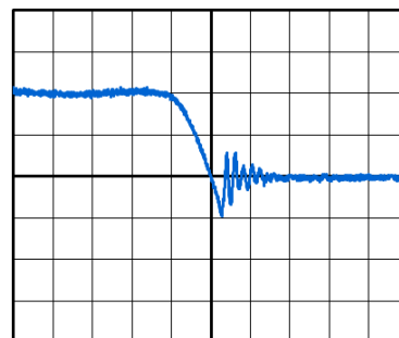
図 2.11 HED リカバリー波形例
