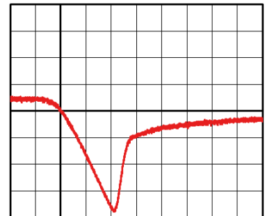
図 2.9 汎用ダイオード t_{rr} 波形例
