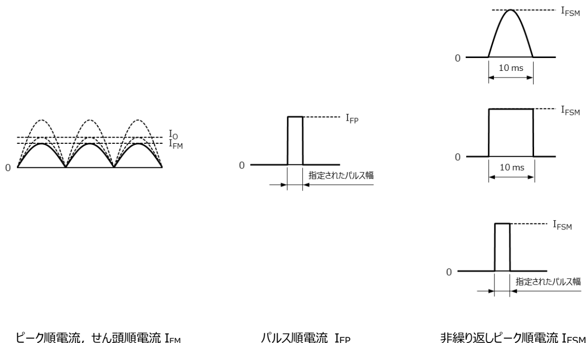
図 1.3 瞬時パルス電流定格の定義
