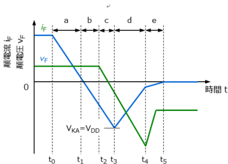
図 2.5 逆回復時間 t_{rr} 波形例
