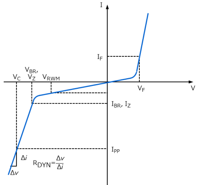
図 2.12 電気的特性の定義
