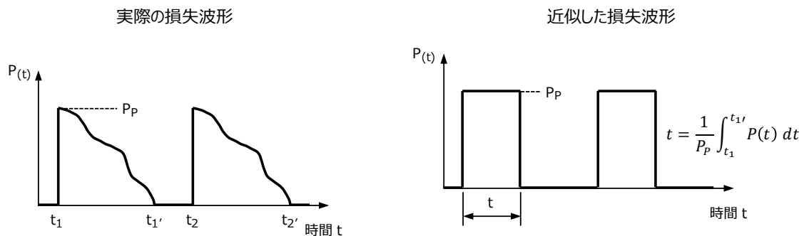
図 2.7 損失波形の近似
