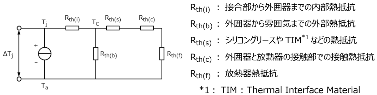
図 2.1 放熱等価回路
