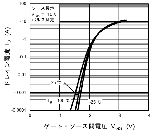
図 7.2 I_D - V_{GS}
