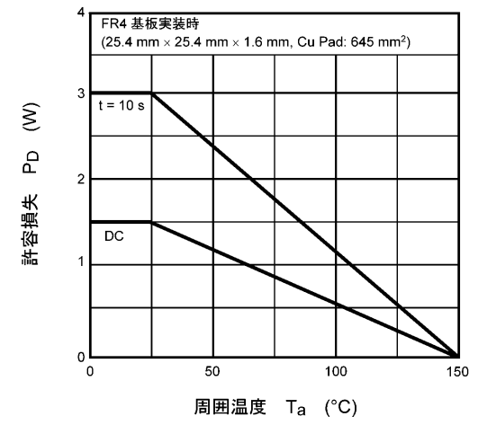
図 7.12 P_D - T_a
