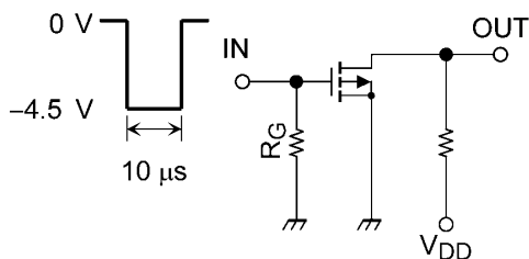
図 5.3.1 スイッチング時間の測定回路
