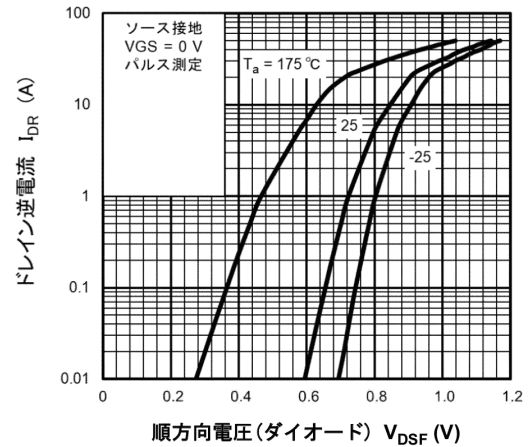
図 8.8 I_{DR} - V_{DSF}
