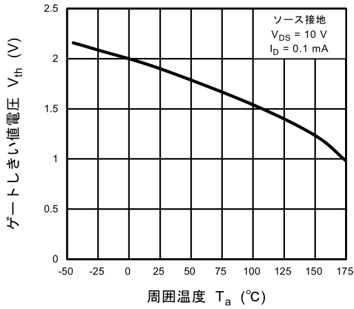
図 7.7 V_{th} - T_a
