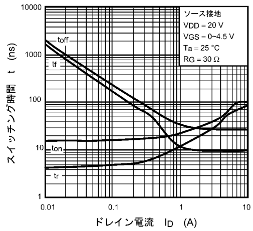
図 7.10 t - I_D
