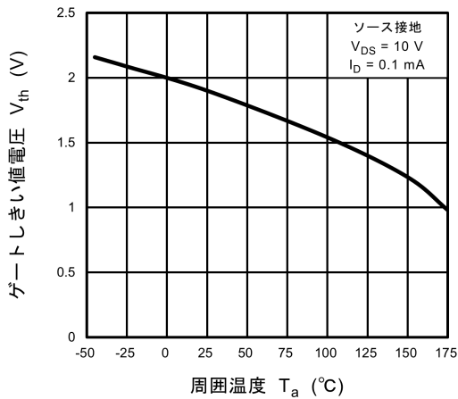
図 8.7 V_{th} - T_a
