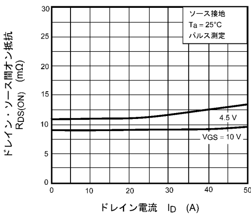
図 7.5 R_{DS(ON)} - I_D
