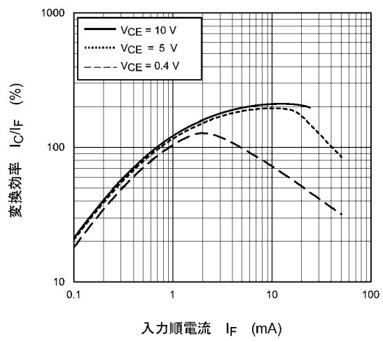
図 11.12 I_C/I_F - I_F
