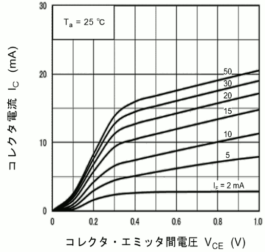
図 11.8 I_C - V_{CE0}
