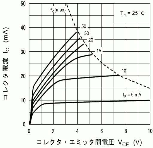
図 11.7 I_C - V_{CE0}
