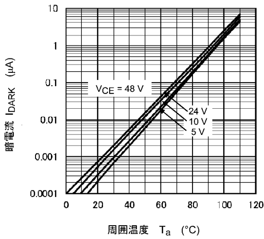
図 11.9 I_{DARK} - T_a
