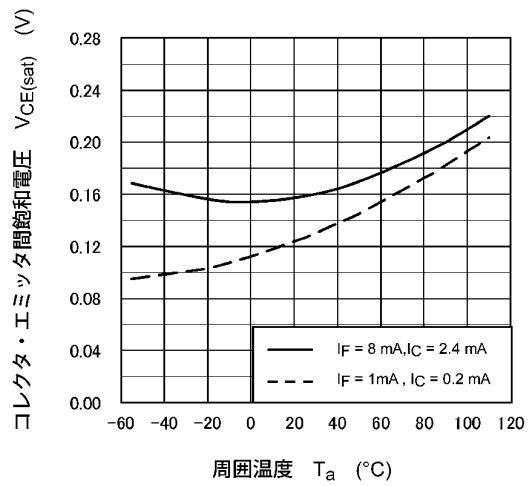
図 11.10 V_{CE(sat)} - T_a
