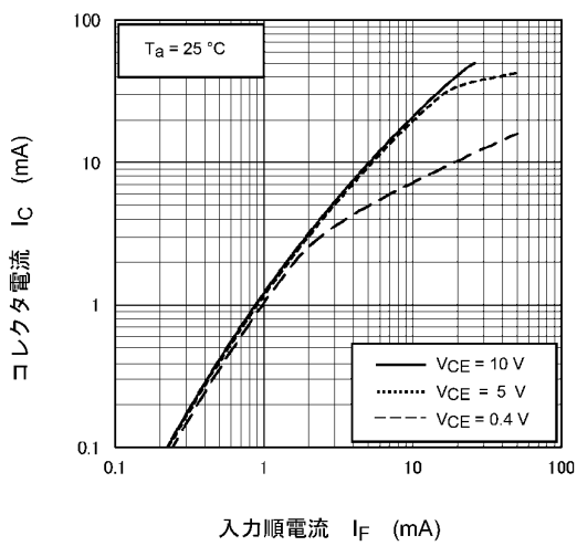
図 11.11 I_C - I_F
