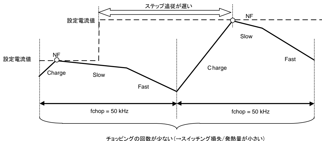
図 4.3 定電流波形 ( f_{chop} = 50 \text{ kHz} の場合)
