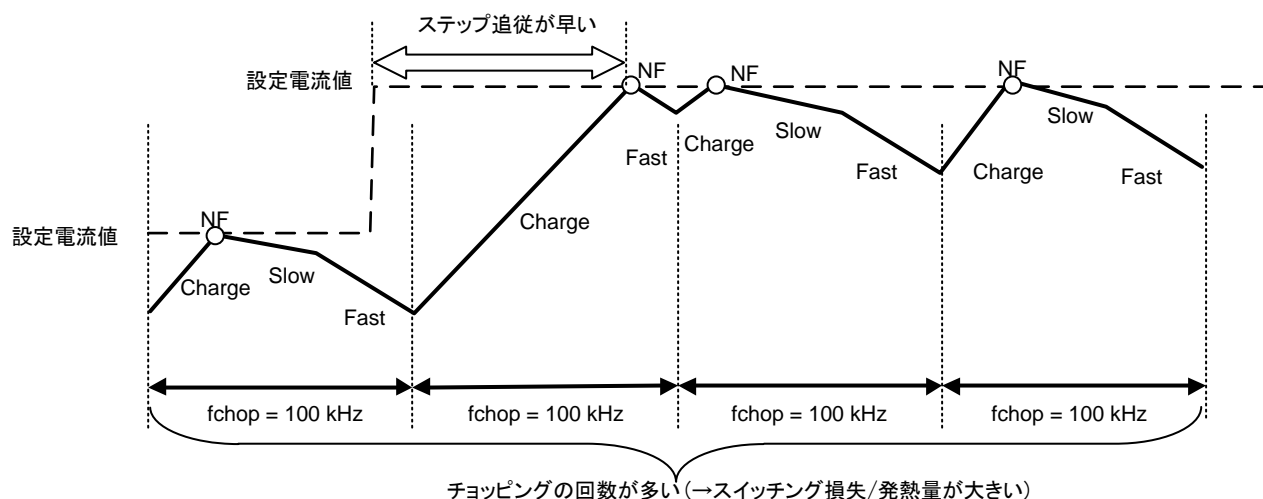
図 4.2 定電流波形 ( f_{chop} = 100 \text{ kHz} の場合)
