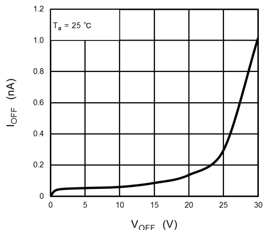
図 12.8 I_{OFF} - V_{OFF}
