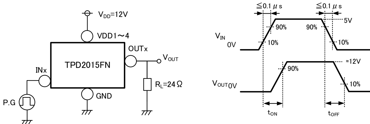
図 11.1 スイッチング時間測定回路
