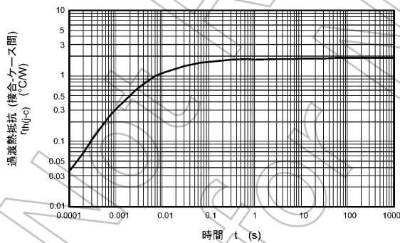
図 9.5 r_{th(j-c)} - t (最大値(保証値))
