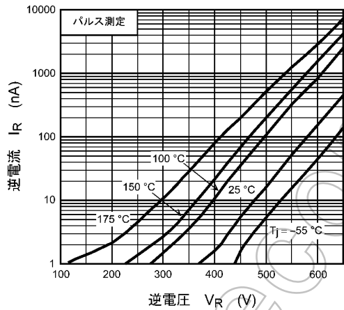
図 9.3 I_R - V_R
